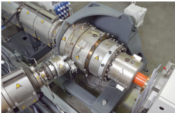
Spider 400-3 die head
